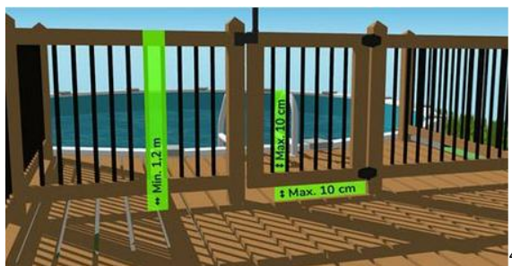
Figure 7 Dimensions exigées pour une enceinte
