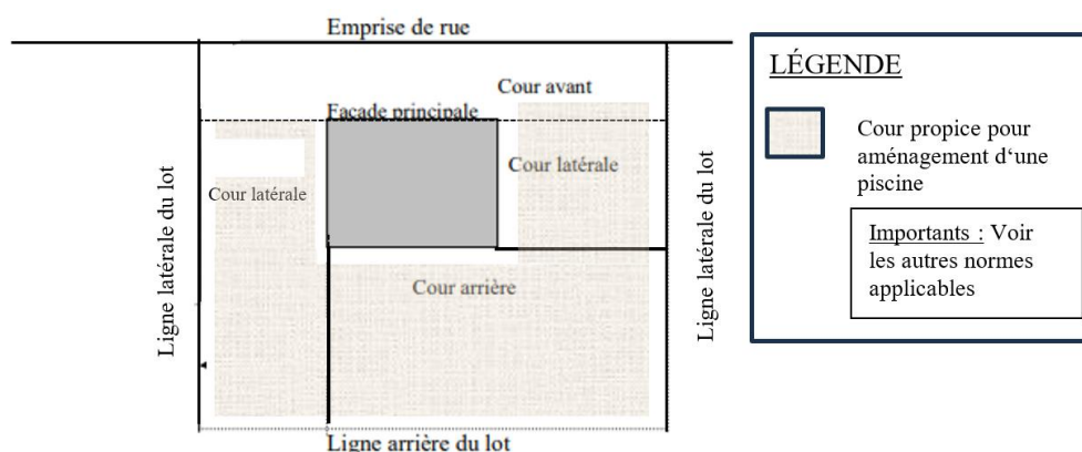
Figure 2 Identification des cours propices pour aménagement d'une piscine et spa sur un terrain intérieur
