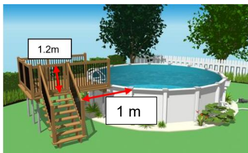
Figure 20 Exemple de plate-forme dont l'accès est protégé par une enceinte
