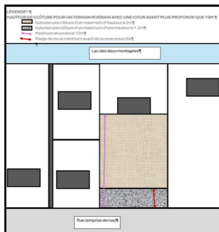
Figure 1 - Clôture pouvant être sur un terrain offrant une cour avant de 15m et plus de profond
